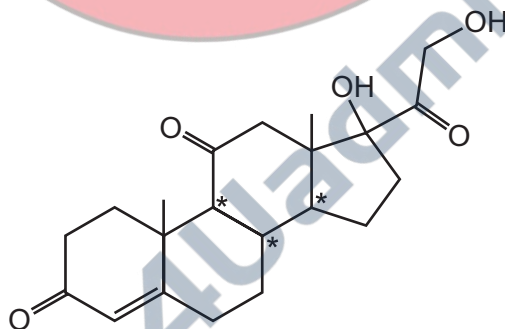
cortisone
